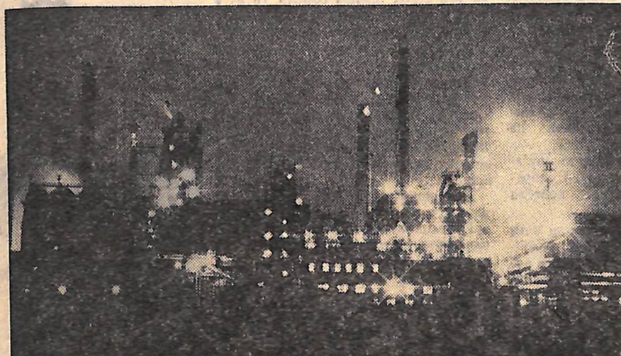
Друга домна під Західно-Сибірського металургійного заводу, яка введена в дію 24 липня цього року, дає чавун. Це найбільша з таких же печей в Сибіру, понад мільйон тонн чавуну буде виплавлятися на ній щорічно.
