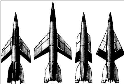
Модели ракет, на которых немецкие ракетчики отработывали форму крыльев в 1942 и 1944 гг.
